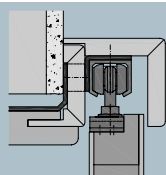
Système en applique: rail, accessoires de guidage, plinthe (habillage du bandeau)
